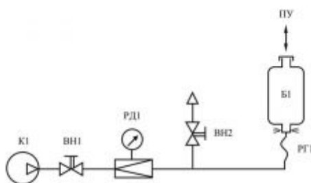
Схема установки для окраски вертикальных трубопроводов. К1 – компрессор (400 л/мин, 8 кг/см 2 ), ВН1, ВВ12 – вентиль шаровый, Ду15, РД1 – регулятор давления с фильтром-клапаном и манометром FR-200 (1500 л/мин, 1/2"), РГ1 – глубокий рукав (Ду9, L = 80 м), Б1 – бачок с форсункой, ПУ – подъемное устройство.
